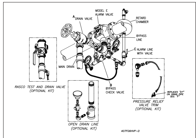
Fig. 8 - E3 Horizontal Trim
